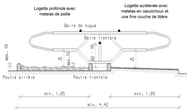
Fig. 2 Logettes opposées respectant les dimensions minimales pour une vache ayant une hauteur au garrot de 135 \pm 5 cm
