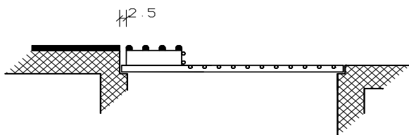
Fig. 11 Grille prolongeant la couche dans une étable à stabulation entravée
