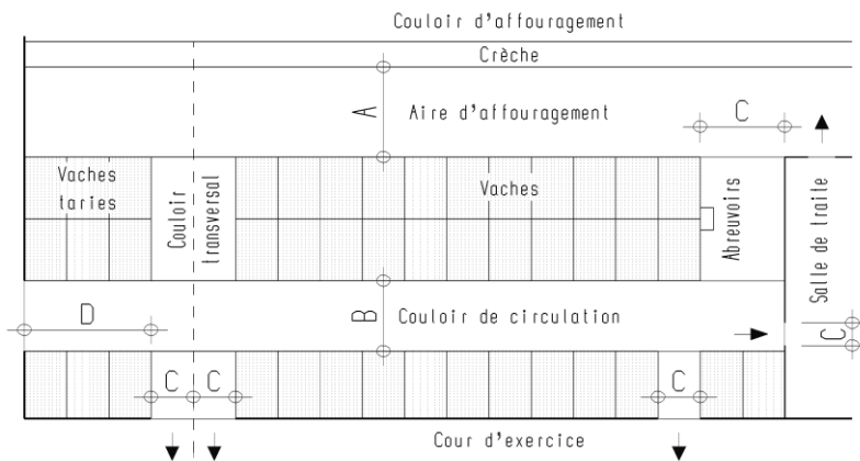
Fig. 3 Dimensions des couloirs d'étable
